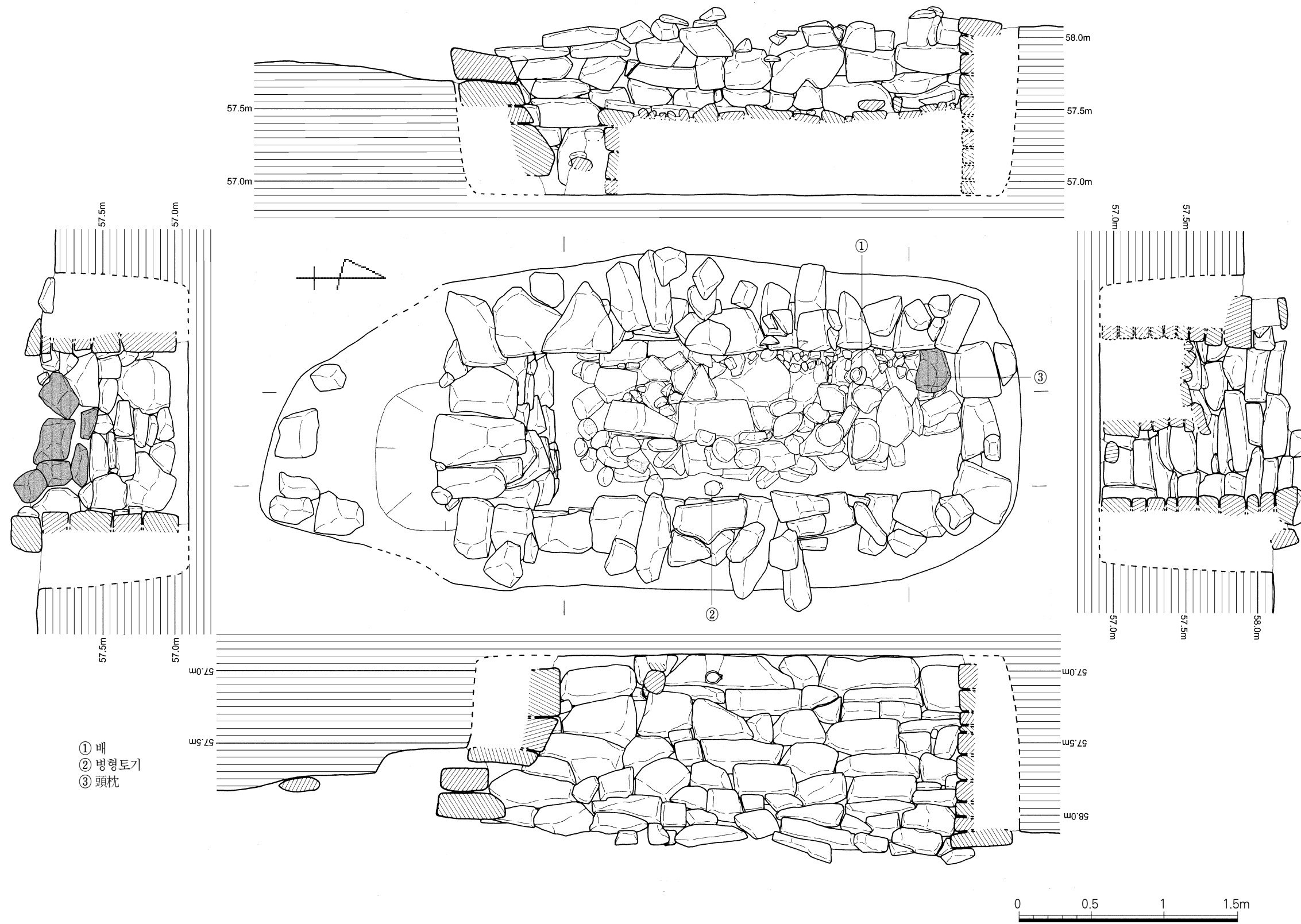
도면 4. 1호 황구식 석실묘
