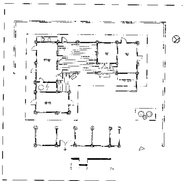
도면 19. 이덕순 가옥 평면도
