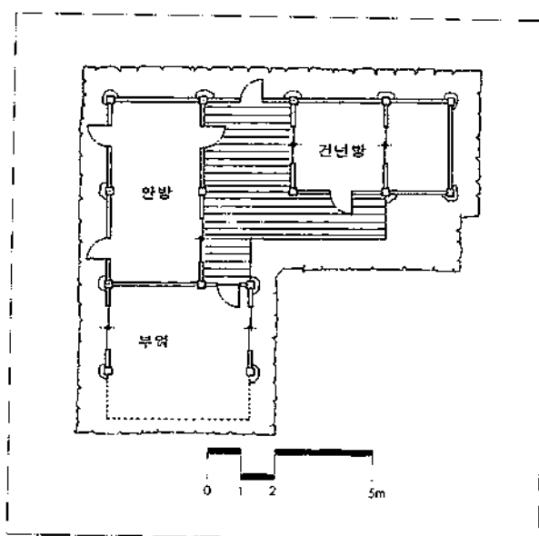
도면 7. 최지숙 가옥 평면도
