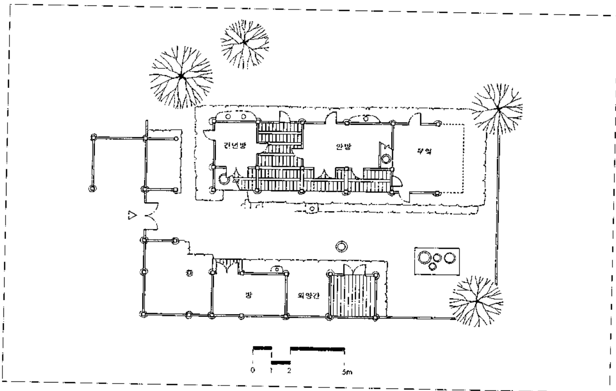
도면 4. 남택수 가옥 평면도
