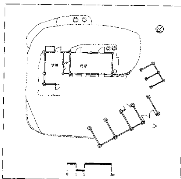
도면 29. 강석규 가옥 평면도
