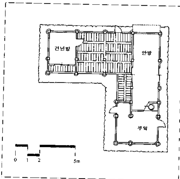
도면 11. 이춘열 가옥 평면도
