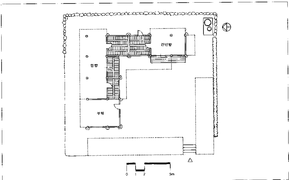
도면 6. 이윤호 가옥 평면도
