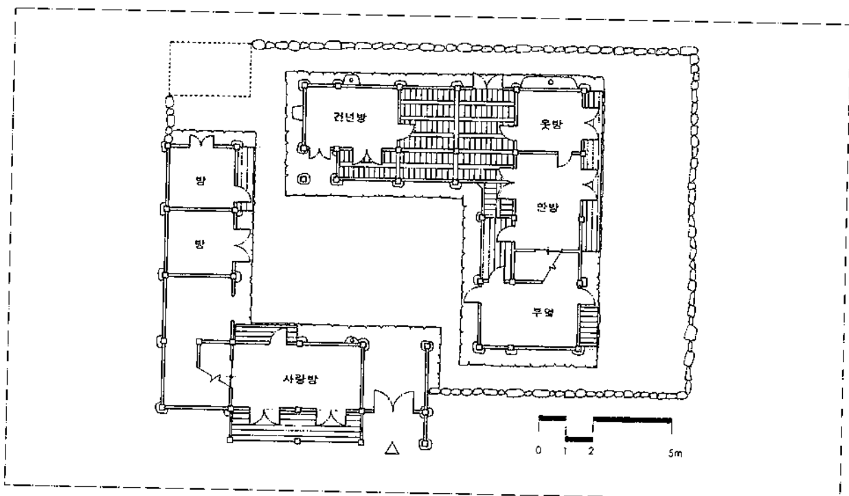
도면 5. 김용학 가옥 평면도
