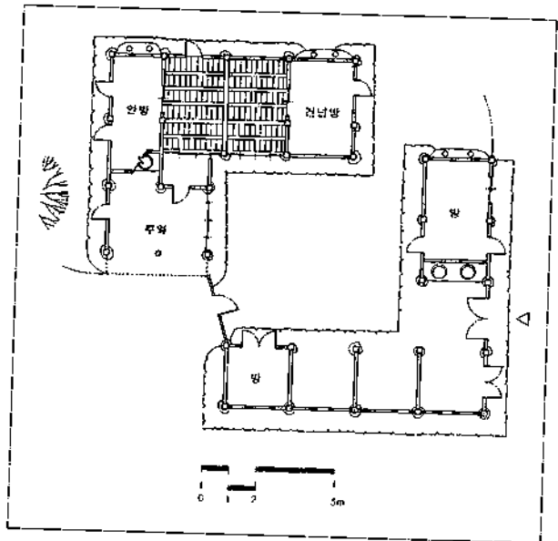
도면 46. 방병식 가옥 평면도
