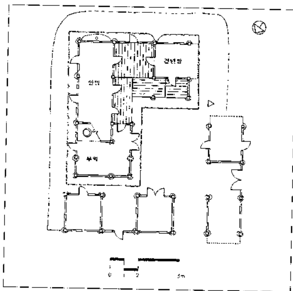
도면 54. 홍성현 가옥 평면도
