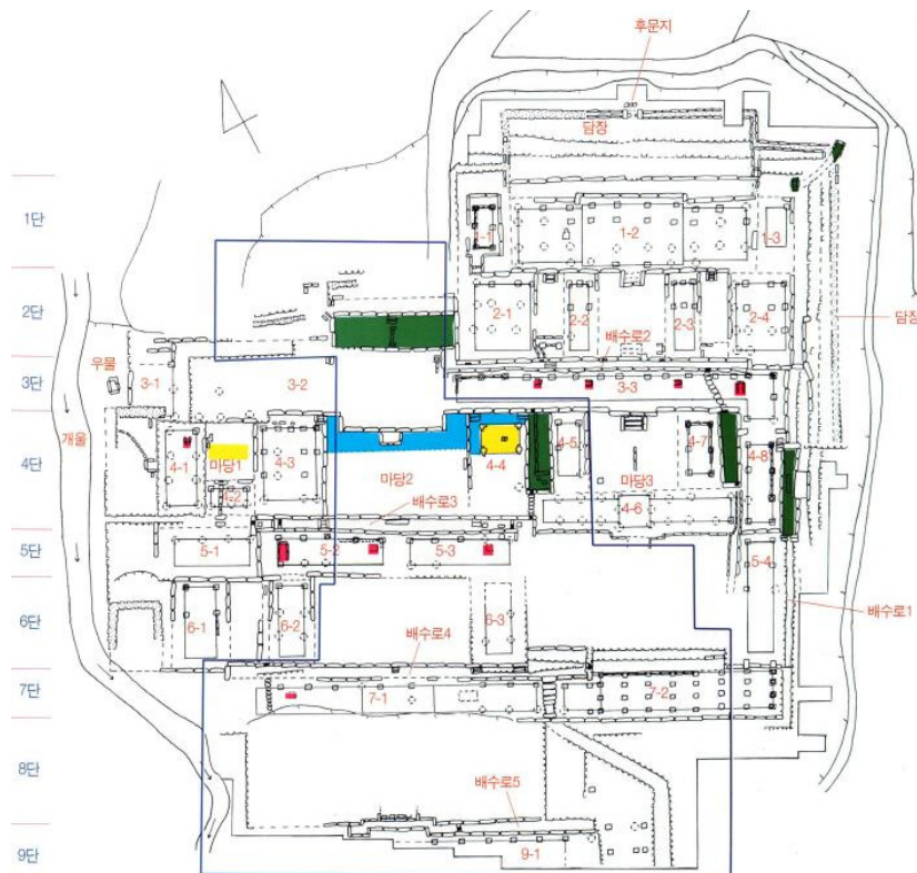
그림 9. 파주 혜음원지 배치도 (단국대학교 매장문화재연구소 2004)
