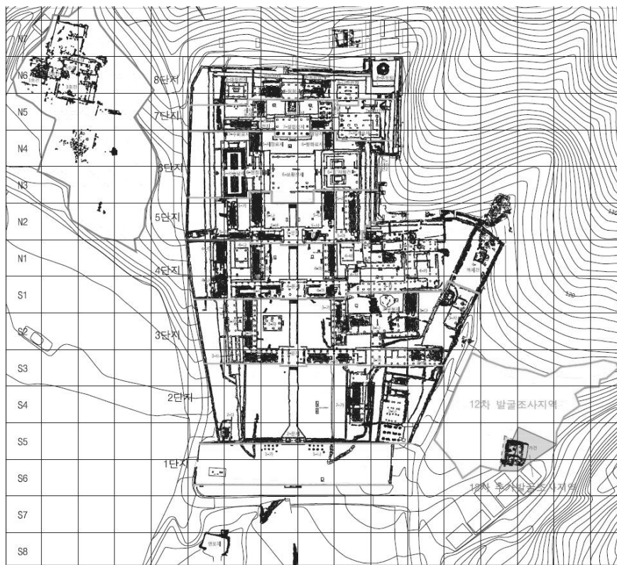
그림 4. 회암사지 배치도 (경기문화재연구원 2017)
